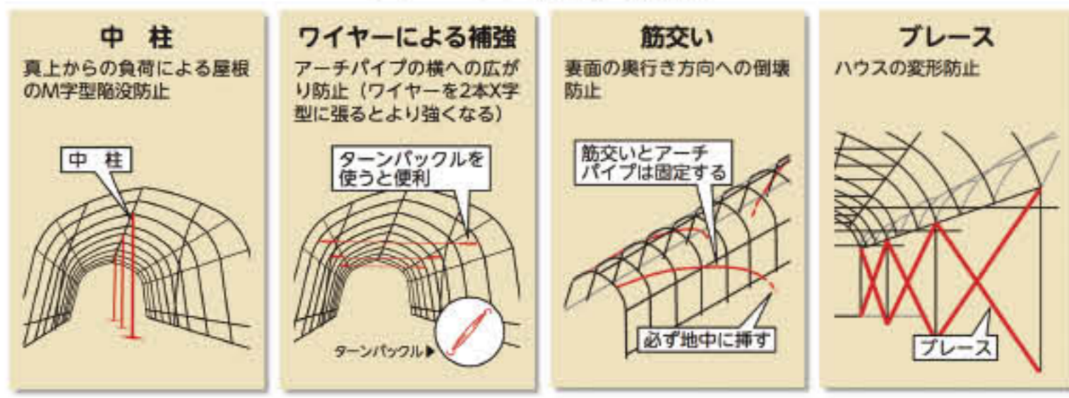
図. ハウス補強の仕方
