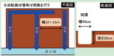
図2 明渠づくり概略(一例)
